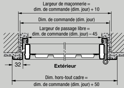
Coupe horizontale
