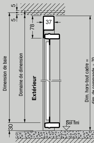
Coupe verticale
